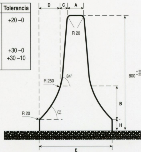
BARRERA DE HORMIGON DOBLE "IN SITU"
