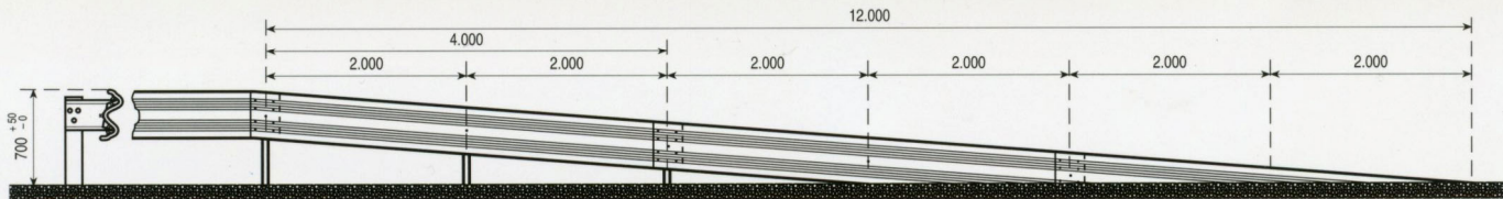
BARRERA METALICA DE SEGURIDAD
