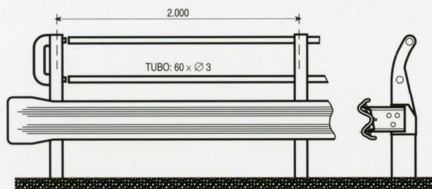
PRETEL METALICO CON BARANDA
