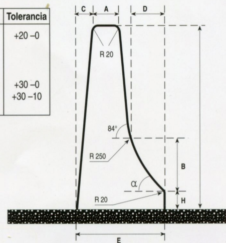
BARRERA DE HORMIGON SIMPLE "IN SITU"
